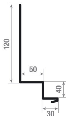
ASTMEGA LIITEPLEKK KLASSIK-profiilile
