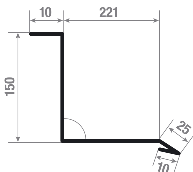
KORSTNAPLEKID
