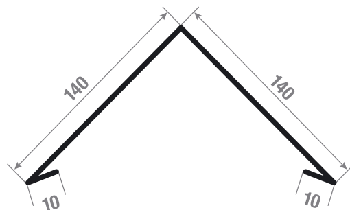
HARJAPLEKK
