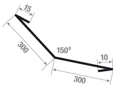
LIITEPLEKK KATUSELT-KATUSELE
