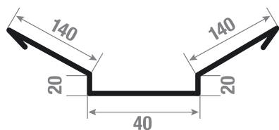
NEELUKATTEPLEKK
