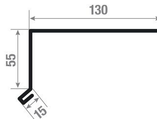
RÄÄSTAPLEKK KLASSIK-profilile
