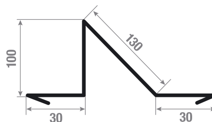
LUMETÖKKEPLAAT
