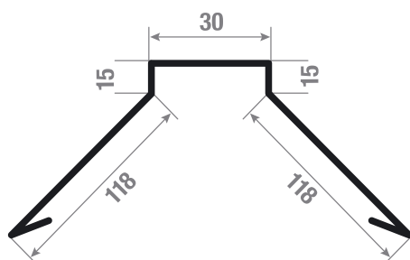
HARJAPLEKK KLASSIK-profiilile
