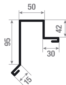
OTSAPLEKK KLASSIK-profiilile
