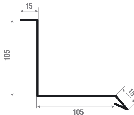
LIITEPLEKK KIVISEINALE
