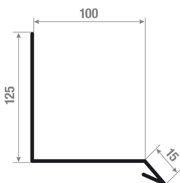
LIITEPLEKK PUITSEINALE
